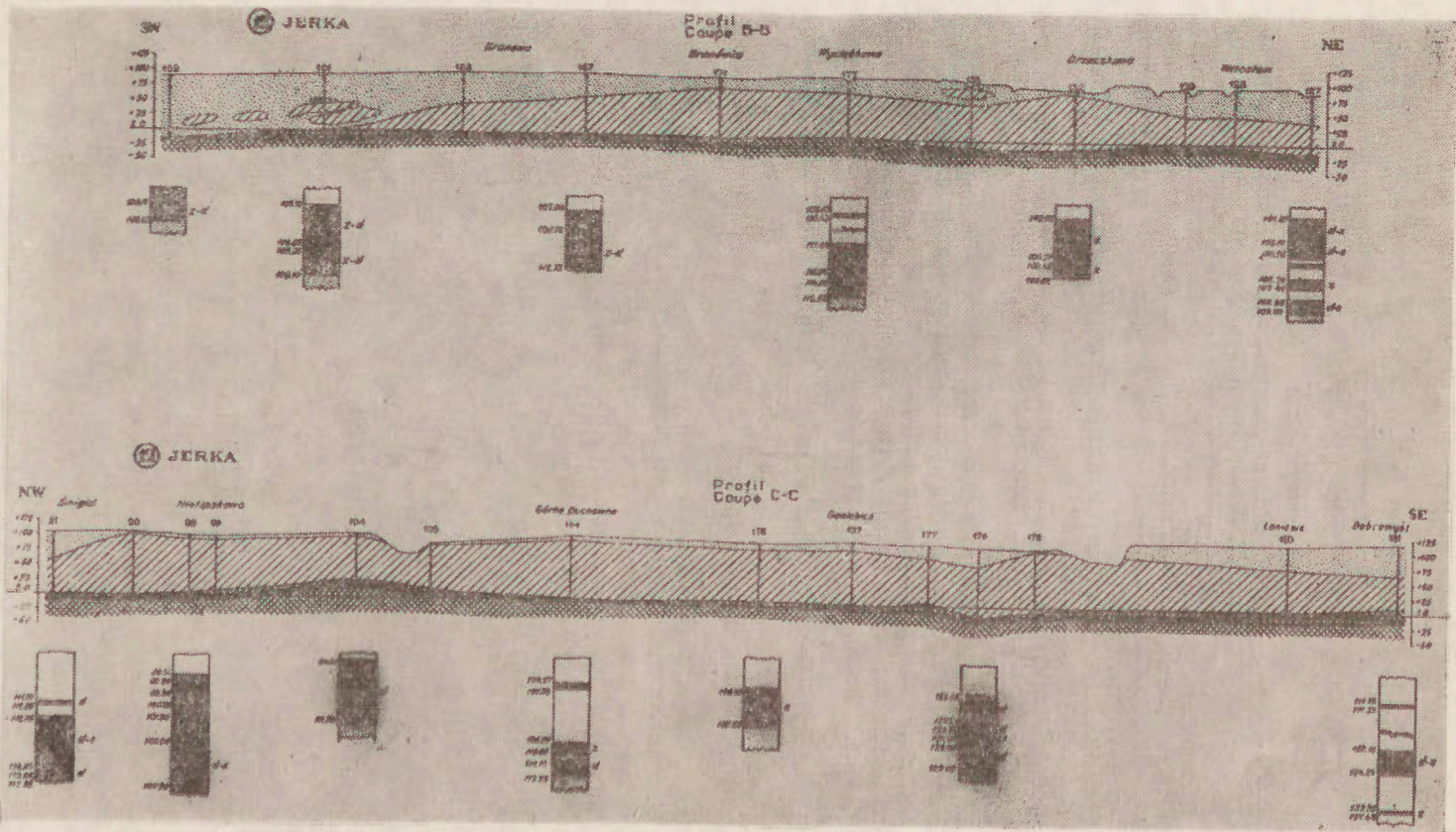
27b. Typowe przekroje geologiczne okolic Jerki (A. Makowski: Węgle brunatne w Polsce, Obszar północno-zachodni), (Fot. J. Skoczylas).
