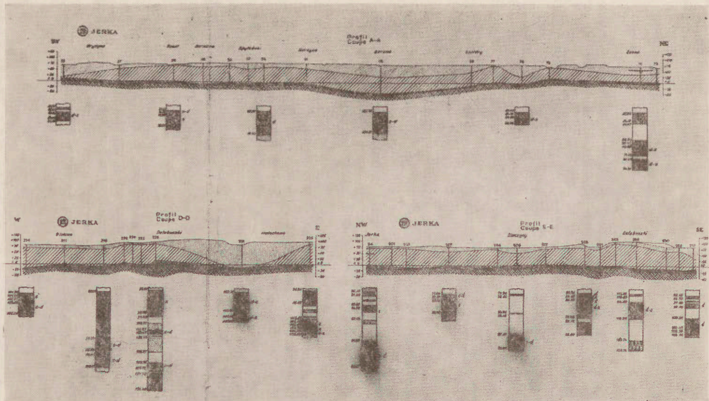
27a. Typowe przekroje geologiczne okolic Jerki. (A. Małowski: Węgle brunatne w Polsce. Obszar północno-zachodni). (Fot. J. Skoczylas).
