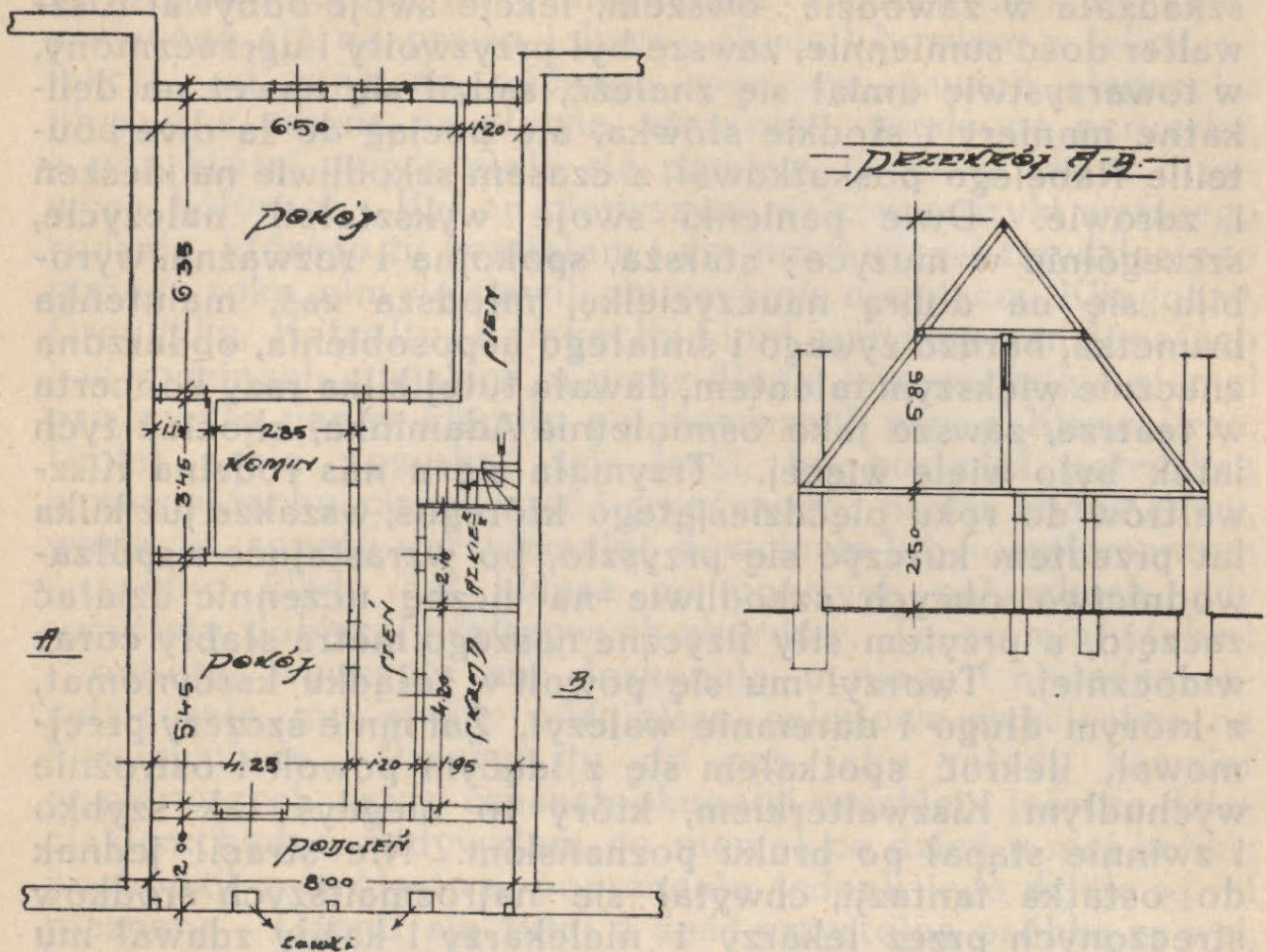
Plan domu z podcieniem w Poniecu.
