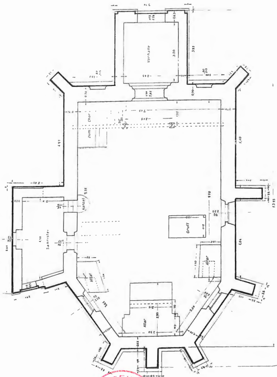
Rzut poziomy kościoła Świętego Krzyża w Kościanie
