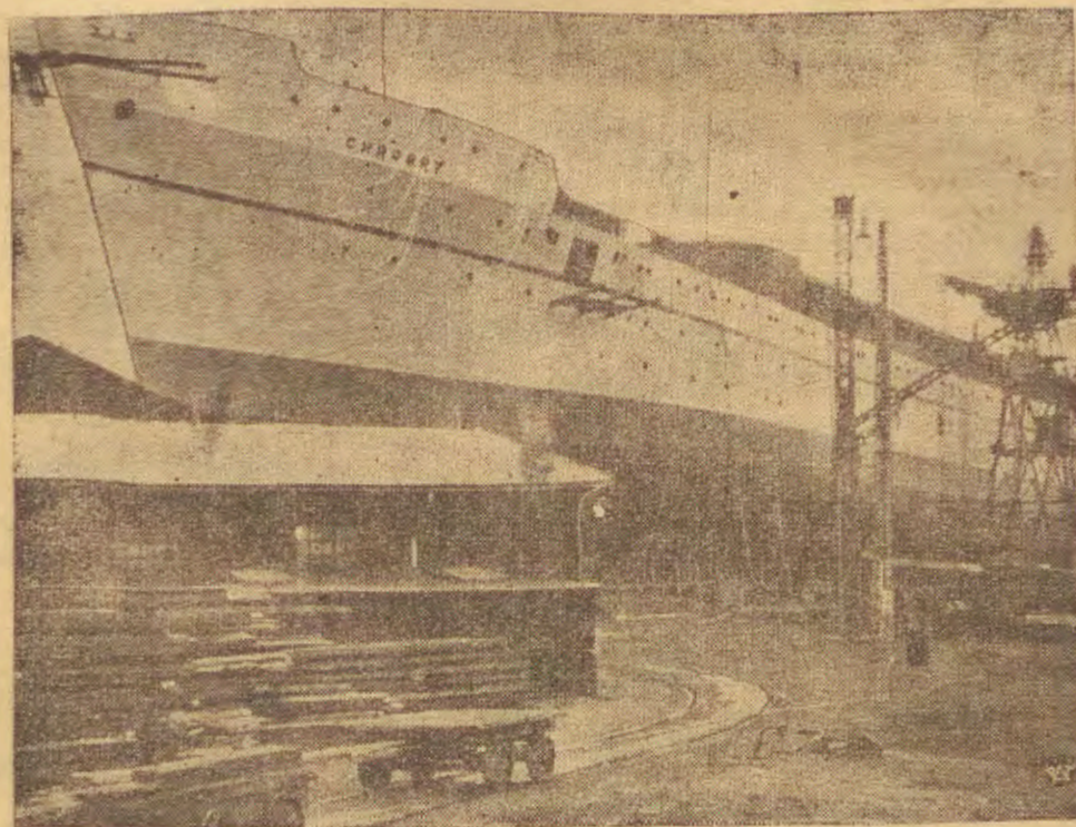
Moment spuszczenia na wodę w duńskiej stoczni w Nakszowie nowego motorowca polskiego M/S „Chrobry“, wykonanego dla linii Gdynia—Ameryka.
