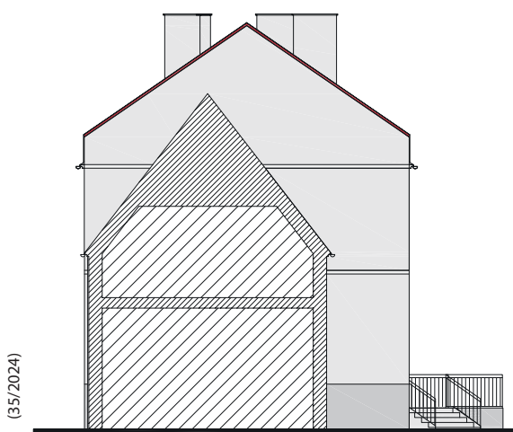
ELEWACJA ZACHODNIA
